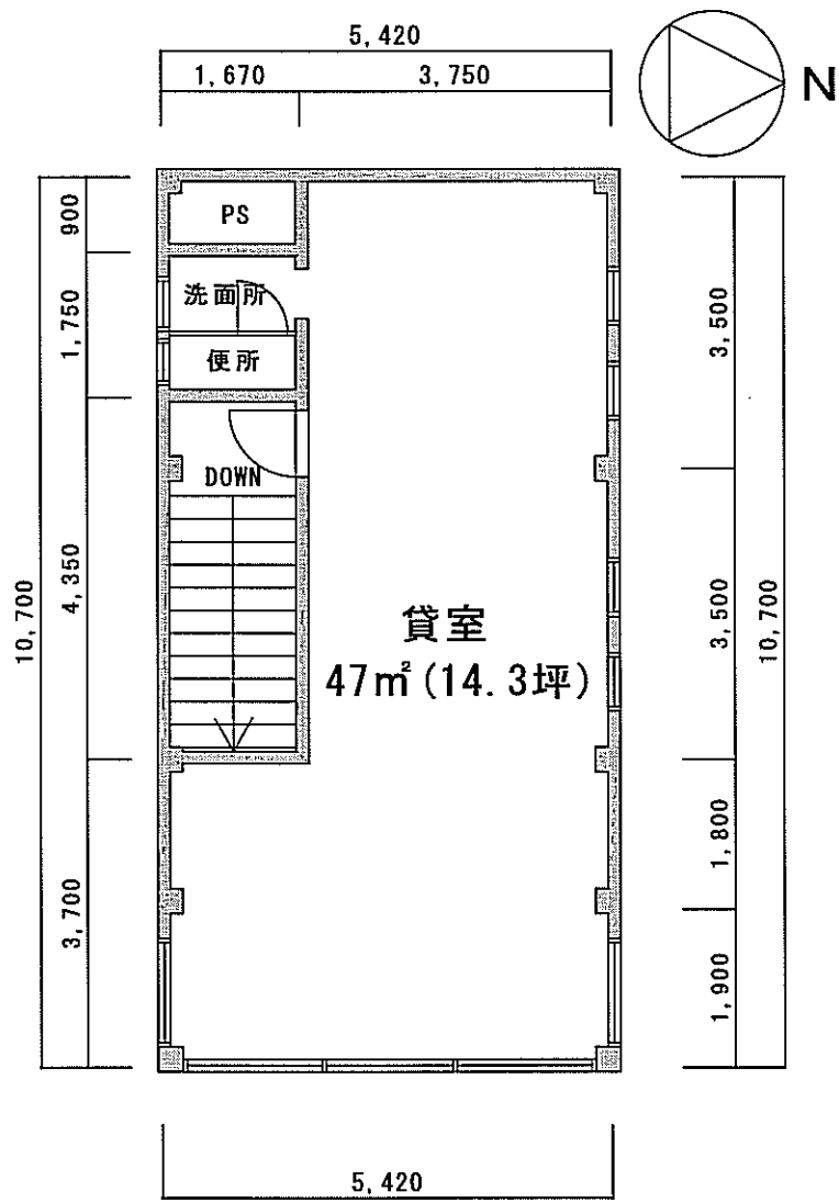
大沢建設第2ビル 3階東平面図 (S=1/100)
