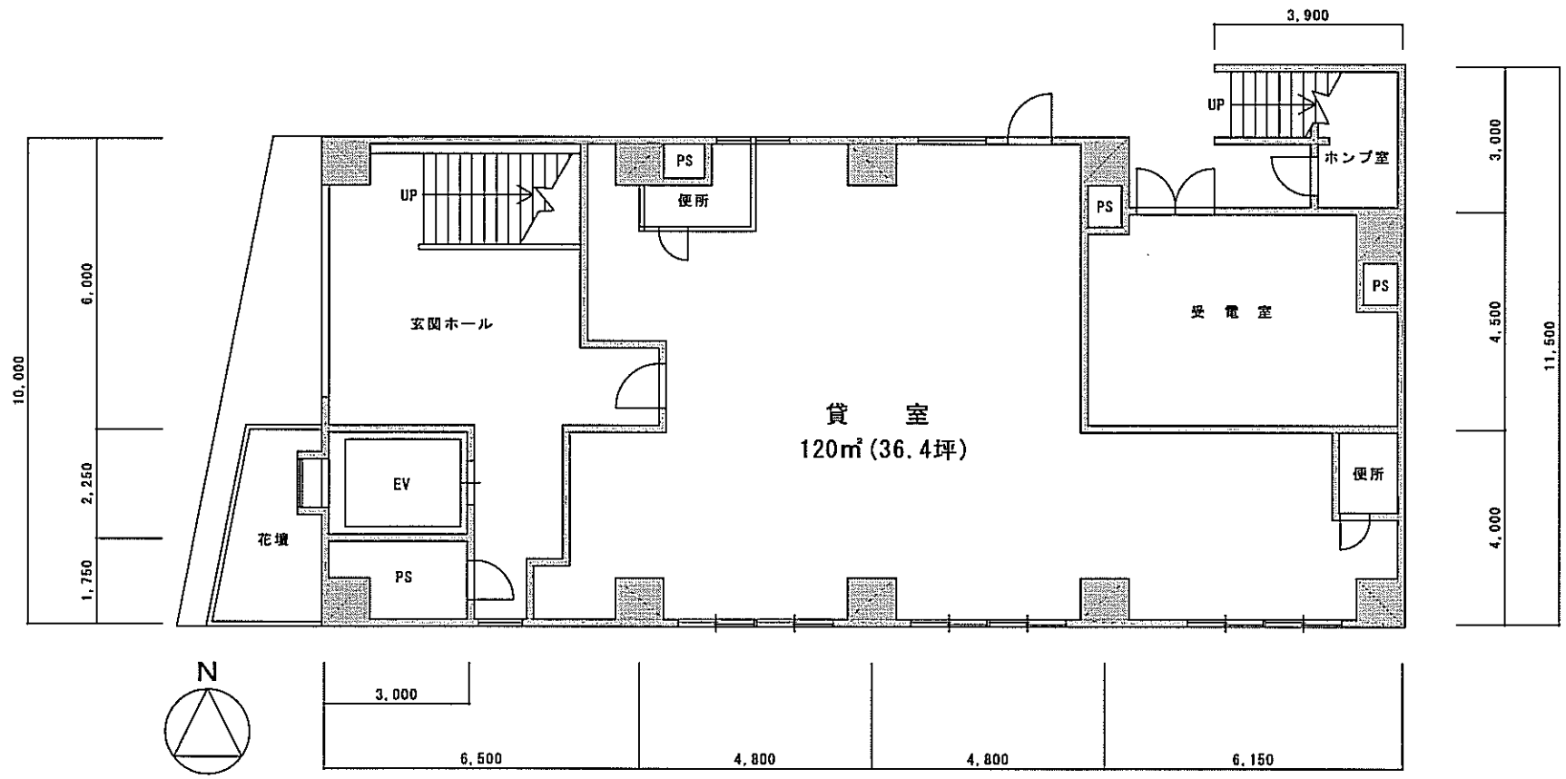
大沢建設第5ビル 1階平面図 (S=1/100)
