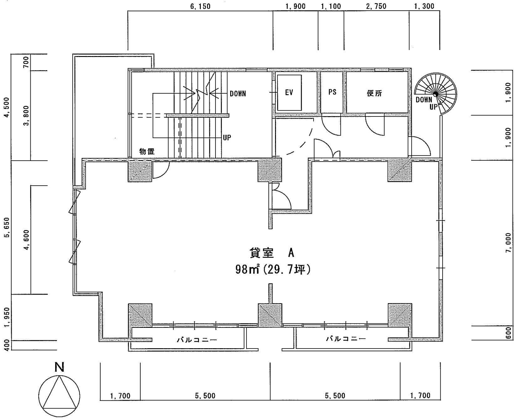
大沢建設第6ビル 2階平面図 (S=1/100)
