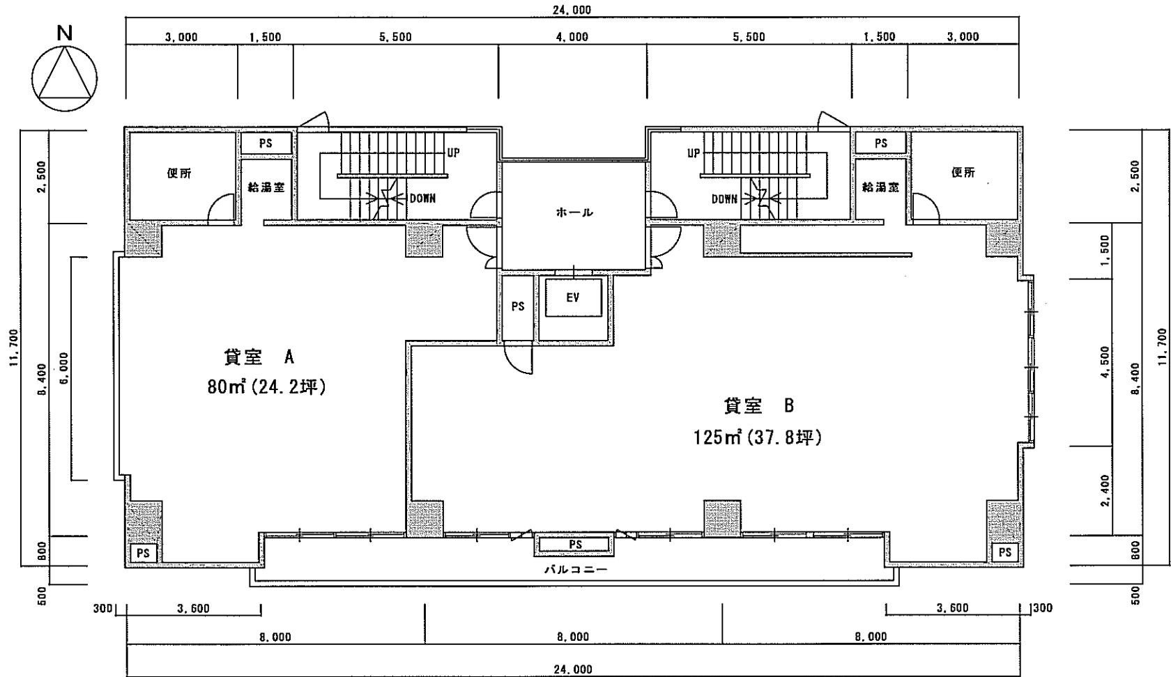
大沢建設第7ビル 8階平面図 (S=1/100)
