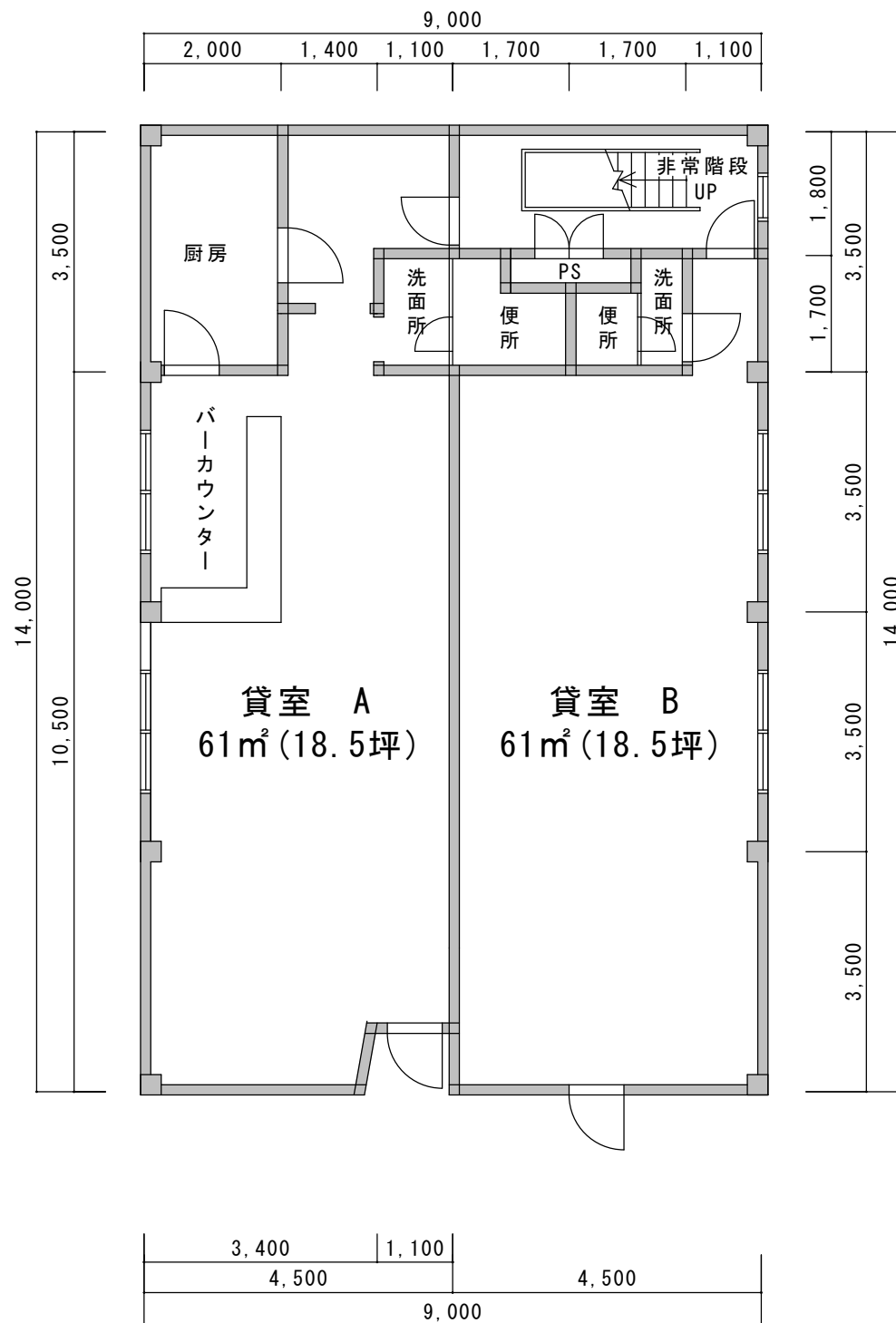
大沢建設第1ビル 間取り例 (S=1/100)
