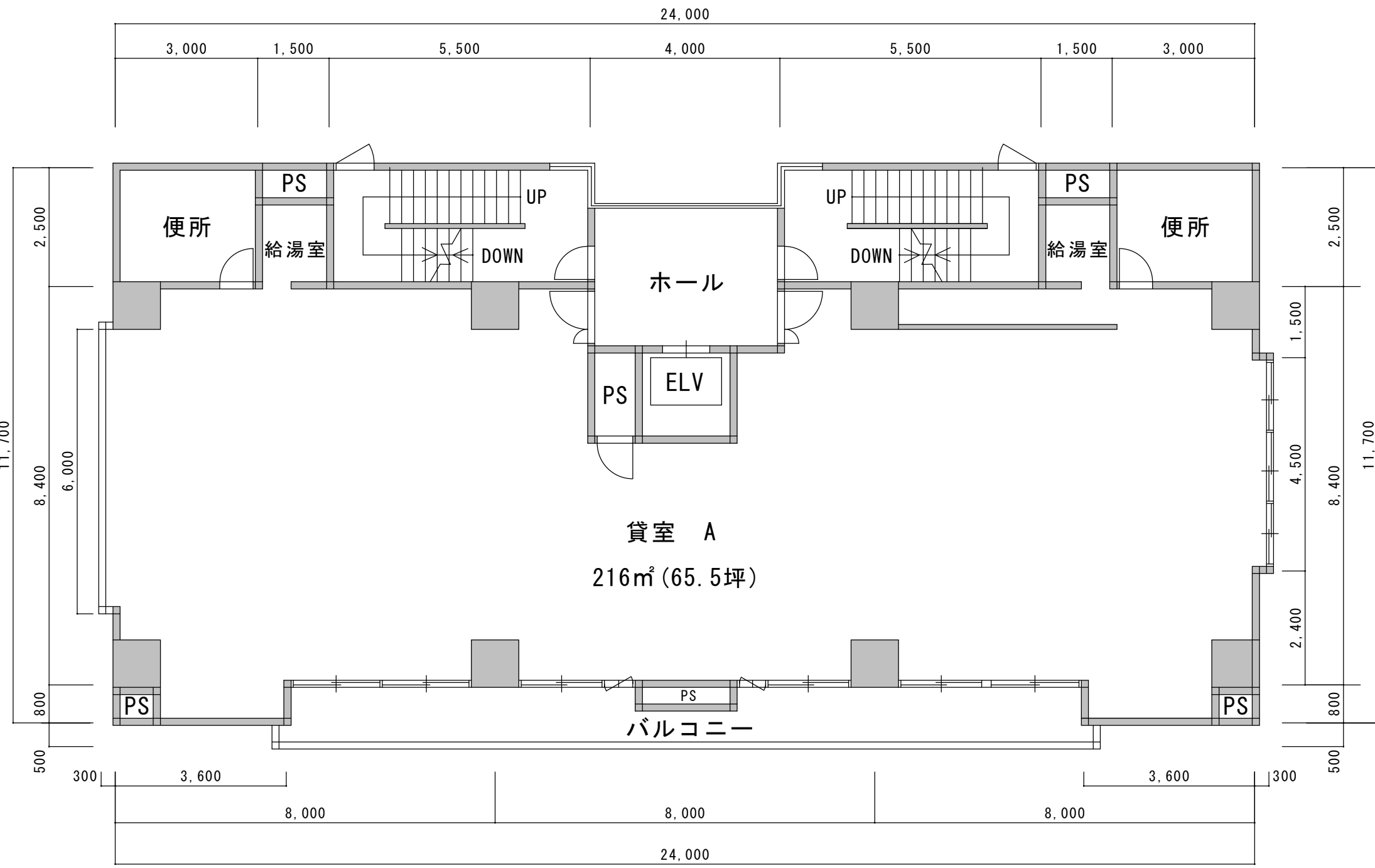
大沢建設第7ビル 間取り例① (S=1/100)
