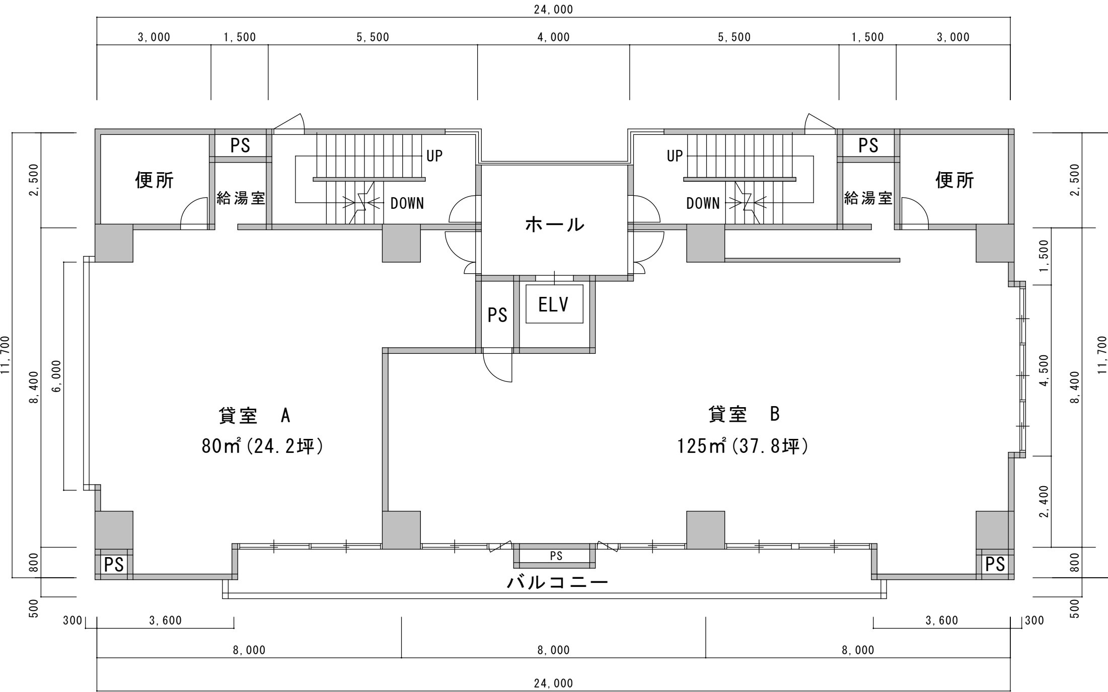
大沢建設第7ビル 間取り例② (S=1/100)
